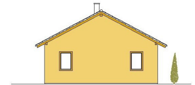
POHLED ZLEVA
