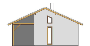
POHLED ZPRAVA
