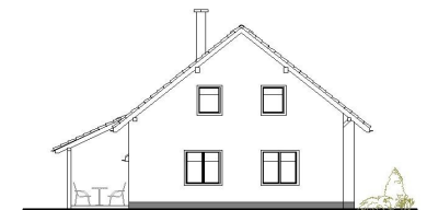
POHLED ZLEVA
