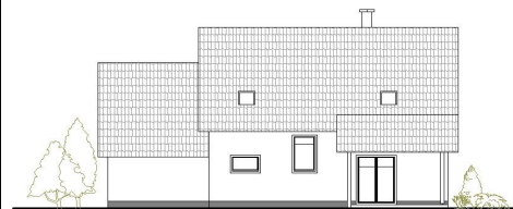
POHLED ZADNÍ
